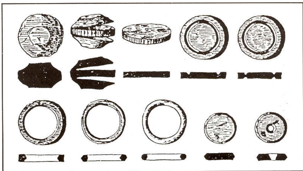
Postup výroby švartnových náramků (podle J. Břeně)
